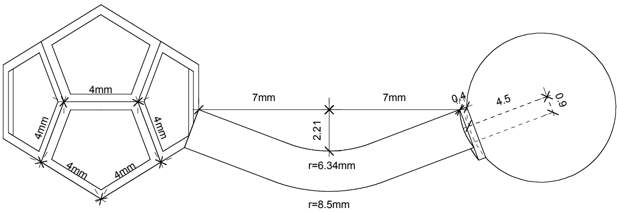
Ansicht 5:1
