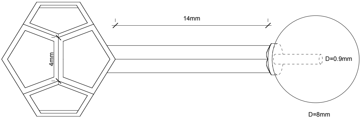
Aufsicht 5:1
